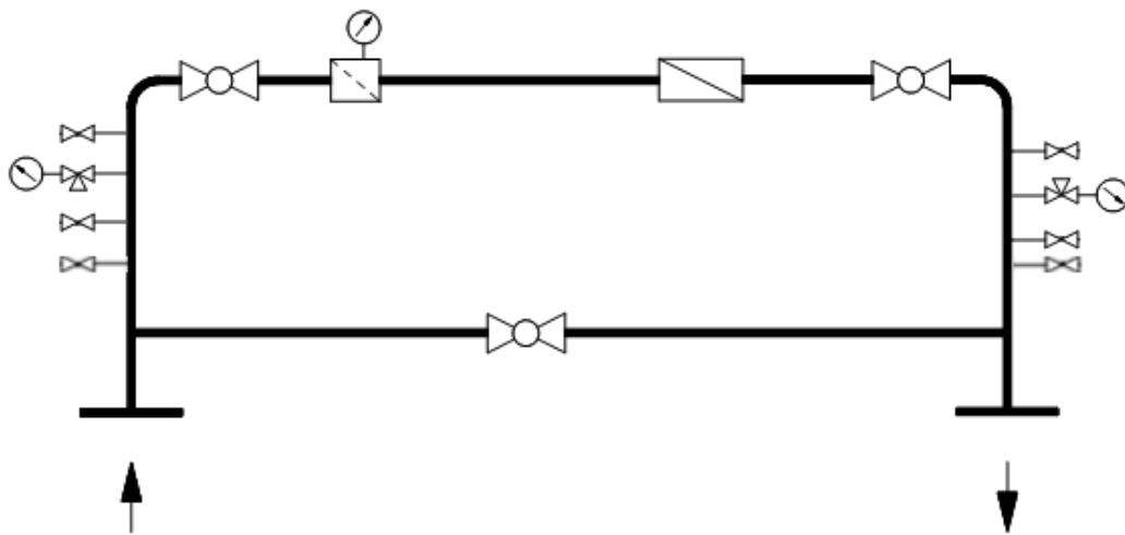
1.1.10. sz. ábra: Mérő állomás
