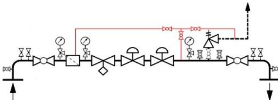
1.1.3. sz. ábra: Egy szabályozóágas, soros kapcsolású kialakítás, kerülő vezeték nélkül
