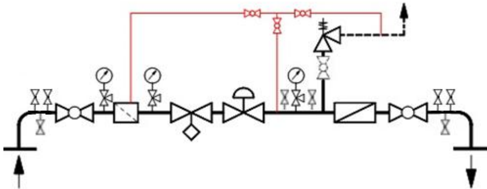
1.1.6. sz. ábra: Egy szabályozóágas, gázmérős kialakítás
