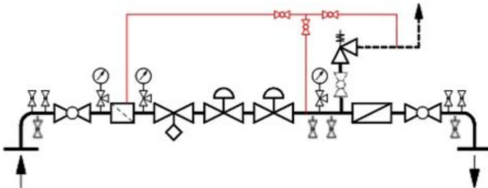
1.1.7. sz. ábra: Egy szabályozóágas, soros kapcsolású, gázmérős kialakítás
