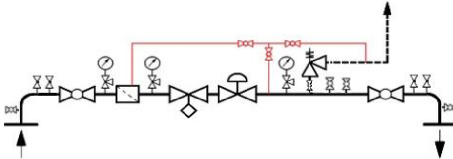
1.1.2. a sz. ábra: Egy szabályozóágas kialakítás, kerülővezeték nélkül
