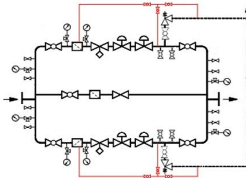
1.1.5. sz. ábra: Két szabályozóágas, vegyes kapcsolású kialakítás
