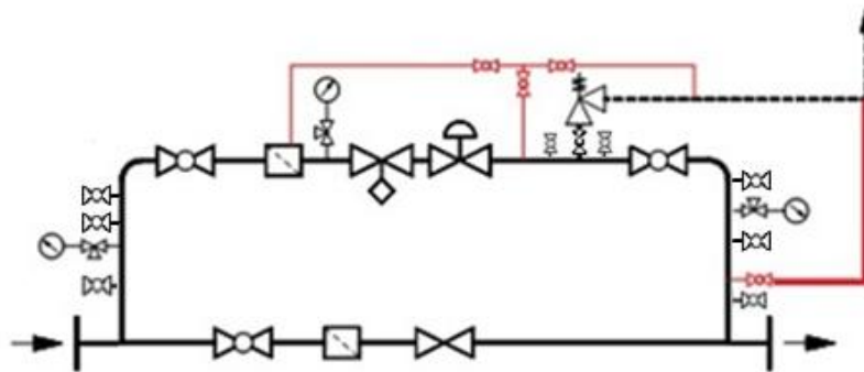
1.1.2. b sz. ábra: Egy szabályozóágas kialakítás, kerülővezetékkel
