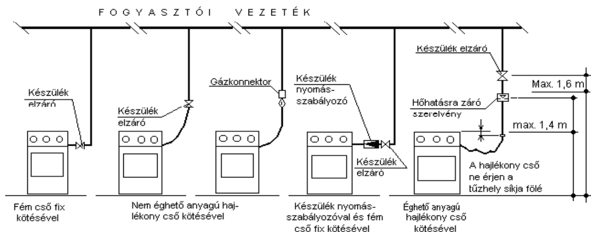
5.2.2. sz. ábra Példa gázfogyasztó készülék elzáró elhelyezésére
