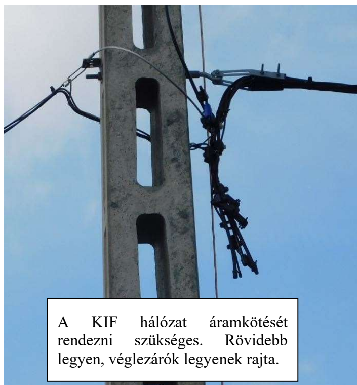
4. Kép KIF áramkötés szigetelt szabadvezetékes hálózaton
