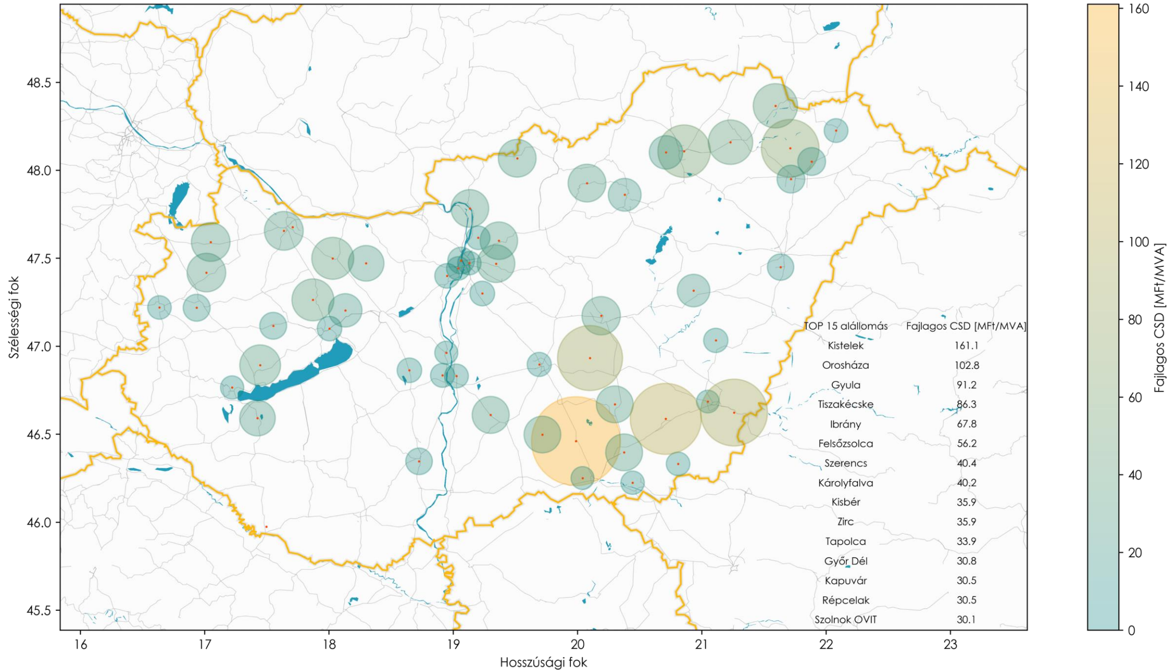
Középfeszültségű hálózatra csatlakozó igények fajlagos közvetett csatlakozási díja a betáplálásra rendelkezésre álló teljesítmény alapján, állomásokra aggregálva; Átlagos CSD: 27.5 M Ft/MVA
