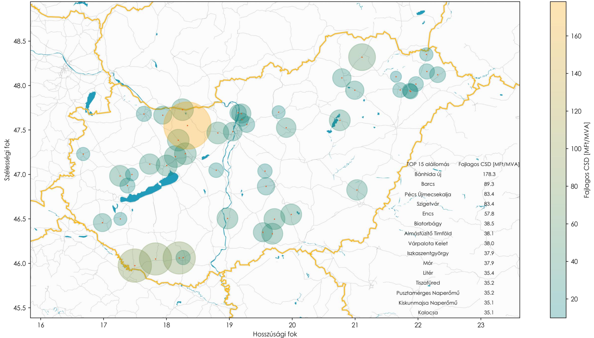
Első közzétételi eljárás keretében jelentkezett, nagyfeszültségű hálózatra csatlakozó igények fajlagos közvetett csatlakozási díja a betáplálásra rendelkezésre álló teljesítmény alapján, alállomásokra aggregálva; Átlagos CSD: 32.9 MFt/MVA
