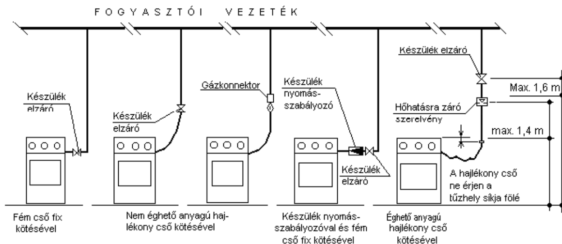
5.2.2. sz. ábra Példa gázfogyasztó készülék elzáró elhelyezésére
