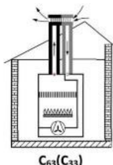
5.2.5.6.8. ábra
