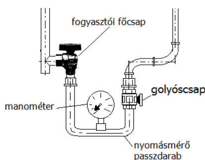
5.4.23 számú ábra Nyomásellenőrző passzdarab elvi ábrája
