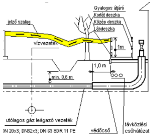
F4) ábrák - Példa jelzőszalag alkalmazására:
