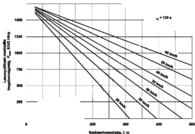
E1.) ábra – Az útszűkületben lebonyolítható forgalom nagyságának meghatározása (120 s periódusidő esetén)
