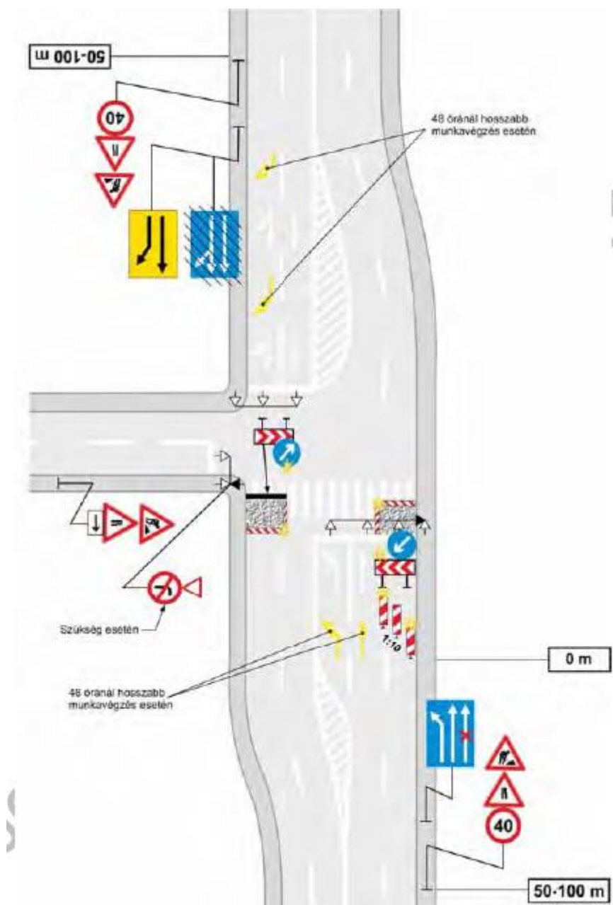
K3. a) ábra – Jelzőlámpás kereszteződés háromütemű átvágása (I. ütem)
