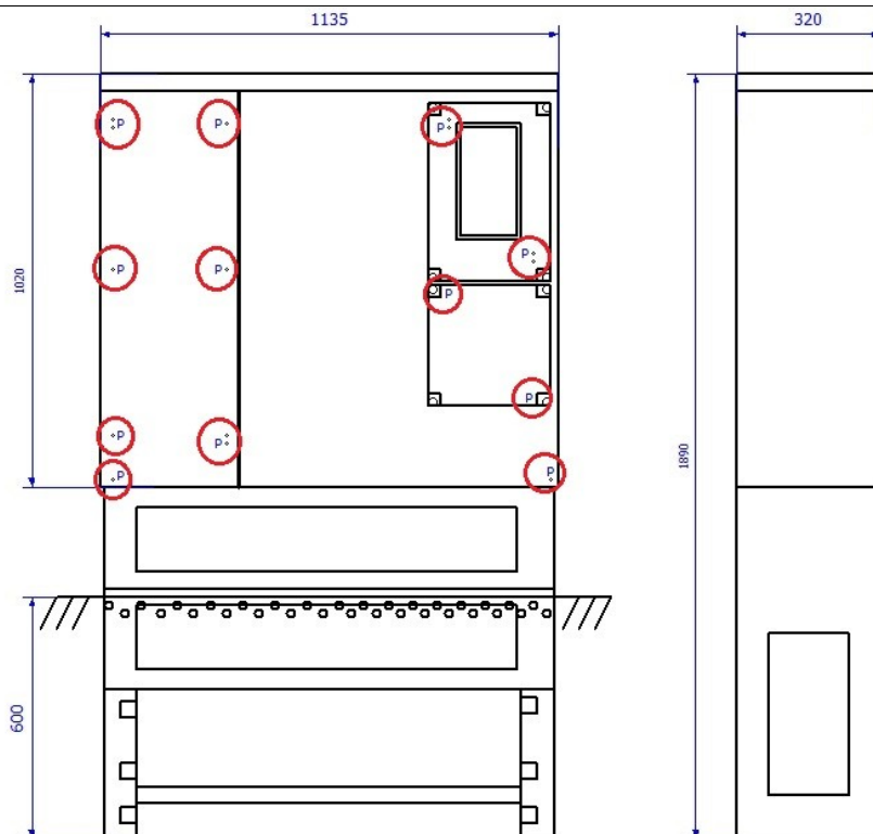
ELRENDEZÉSI RAJZ PLOMBÁLÁSI HELYEKKEL:
