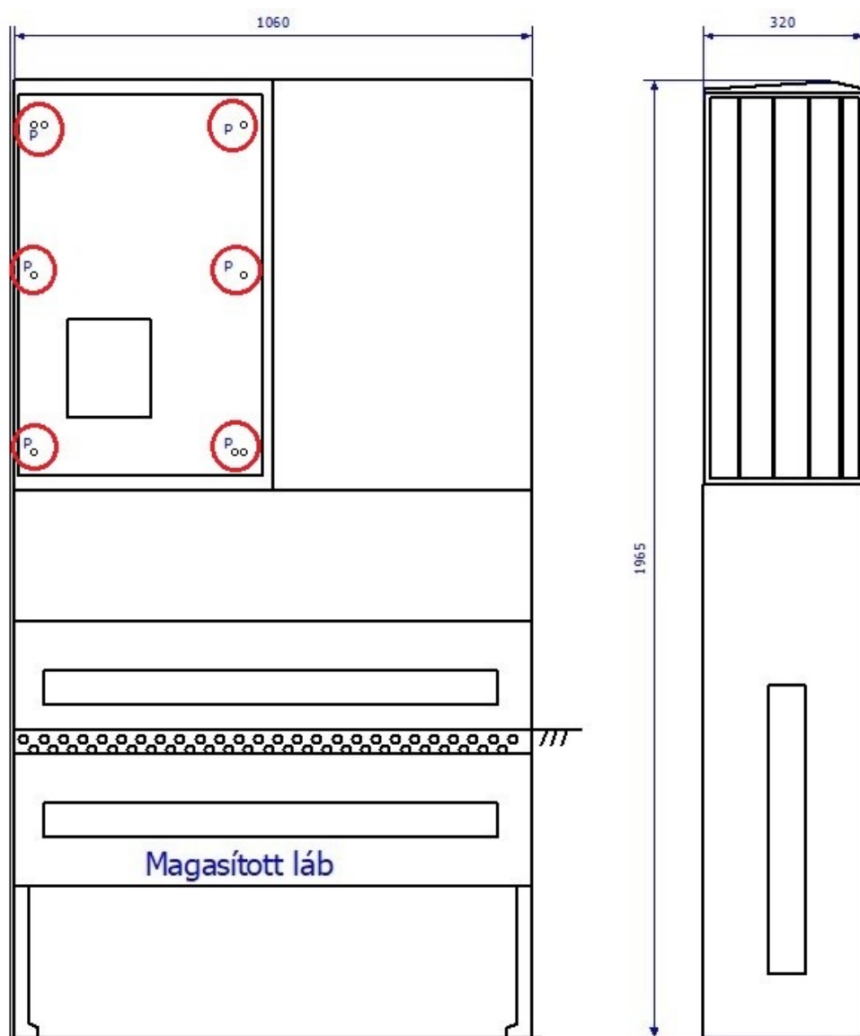
ELRENDEZÉSI RAJZ PLOMBÁLÁSI HELYEKKEL:
