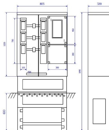
KÖRVONALRAJZ:
