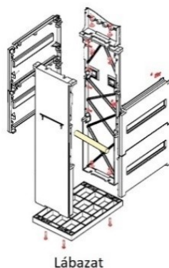
Lábazat
