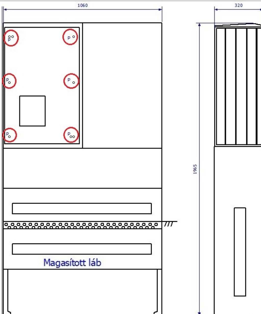
ELRENDEZÉSI RAJZ PLOMBÁLÁSI HELYEKKEL:
